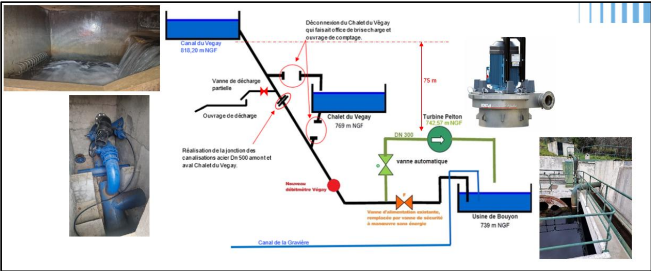
Investissement contractuel - Travaux de pose de la microturbine – Usine de potabilisation (Bouyon) – Schéma de principe
